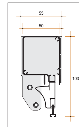
Cassonetto, barra maniglia e cuffia
