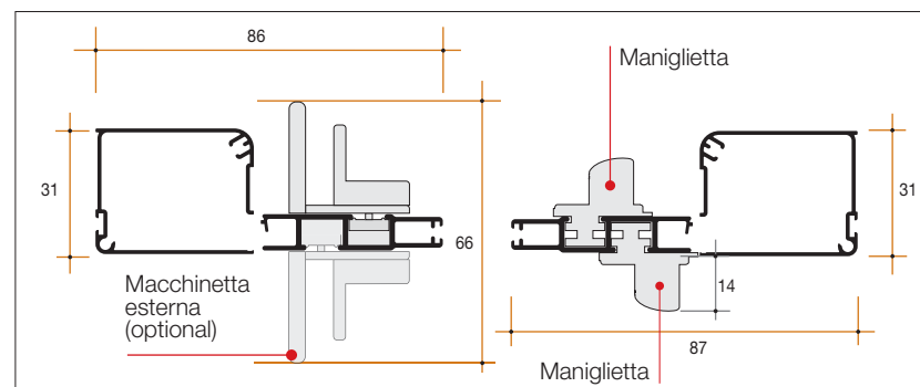
Ingombri versione a due battenti
