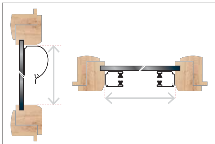
Misure foro/luce
