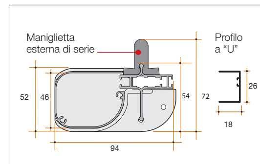
Ingombri versione a due battenti
