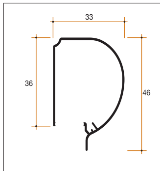
Misure foro/luce
