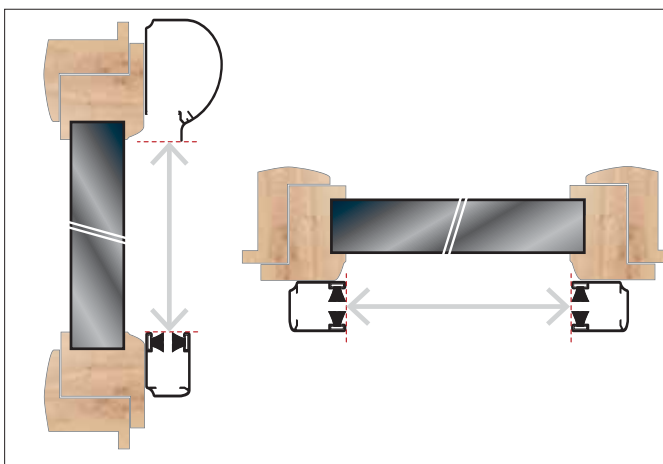
Misure vetro (Solo per versione attacco frontale)
